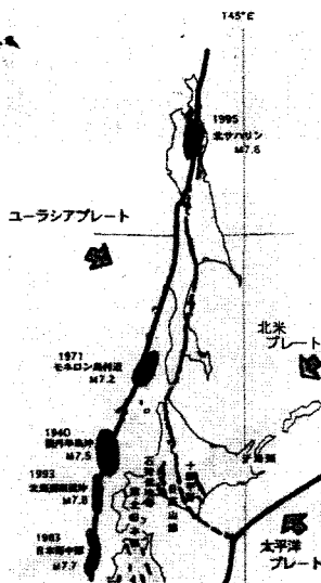
図1 北海道周辺のプレート境界と日本海側の大地震
